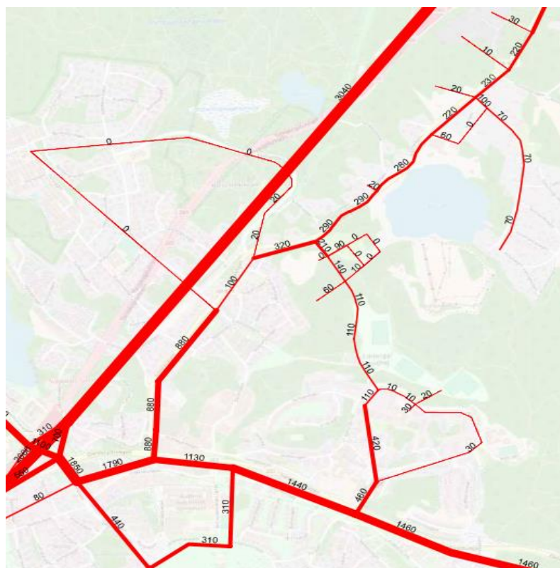
Figur 11. De modellerade trafikflödena under eftermiddagens maxtimme år 2020.
