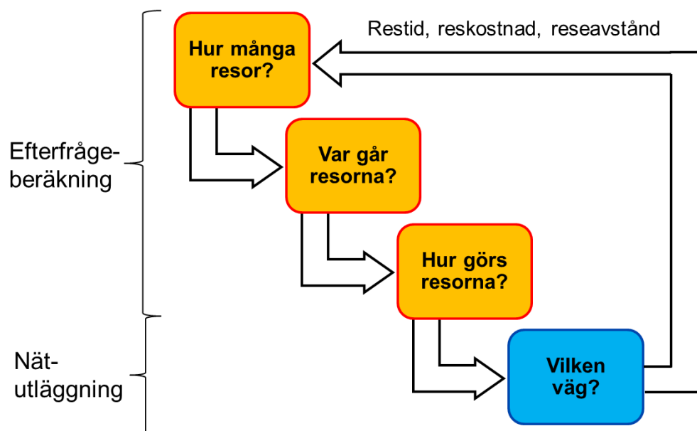
Figur 3. LuTrans struktur.
